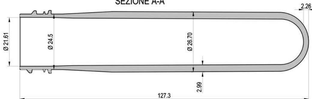
SEZIONE A-A
